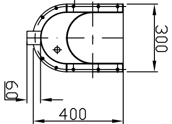
SEZ.A-A
