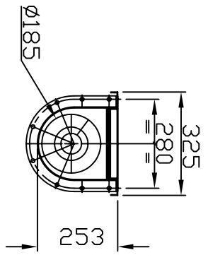
SEZ.C-C
